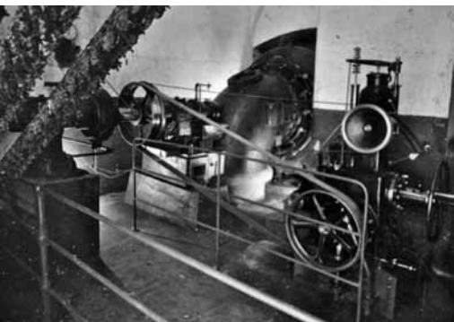
Turbina de la fàbrica Tèxtil Martí, Llopart y Trenchs, SA, d'Alcanís de Rosselló, els anys 1940
