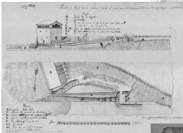
Plànol de reforma del Canal de Pinyana vora el molí fariner d' Alfarràs, l'any 1820
