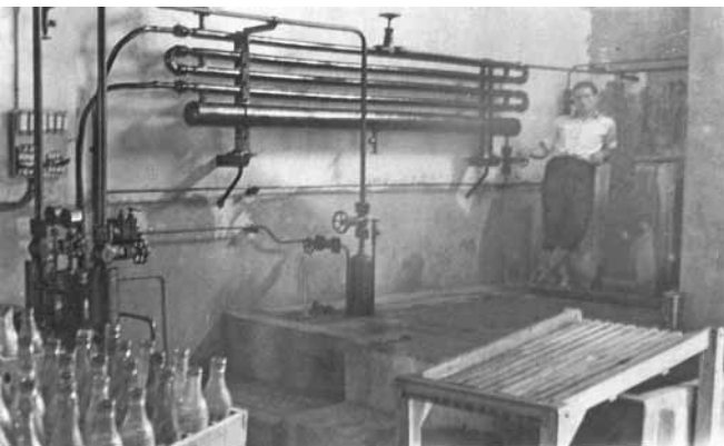
Estructura del circuit de tubs i aparells complementaris emprada en la producció de gel industrial per l'empresa Carbónicas M. Llorens , d'Almenar, de l'any 1958
