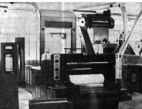
Equipaments de la secció de teixit de la fàbrica Mata y Pons , de la Mata de Pinyana, l'any 1970
