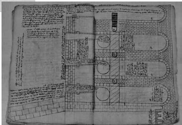
El molí de Regolf d'Almenar, segons el plànol per la seva construcció l'any 1543
